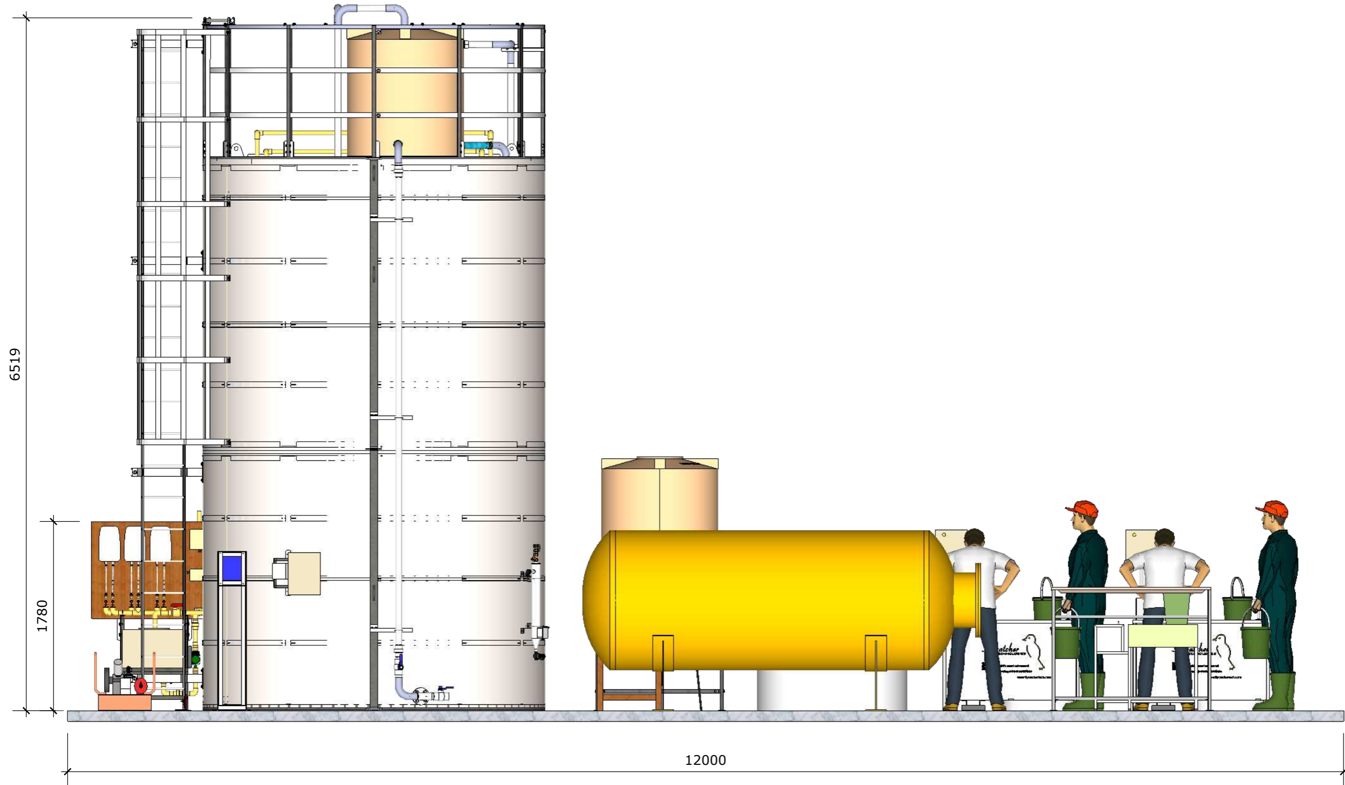
ELEVATION
