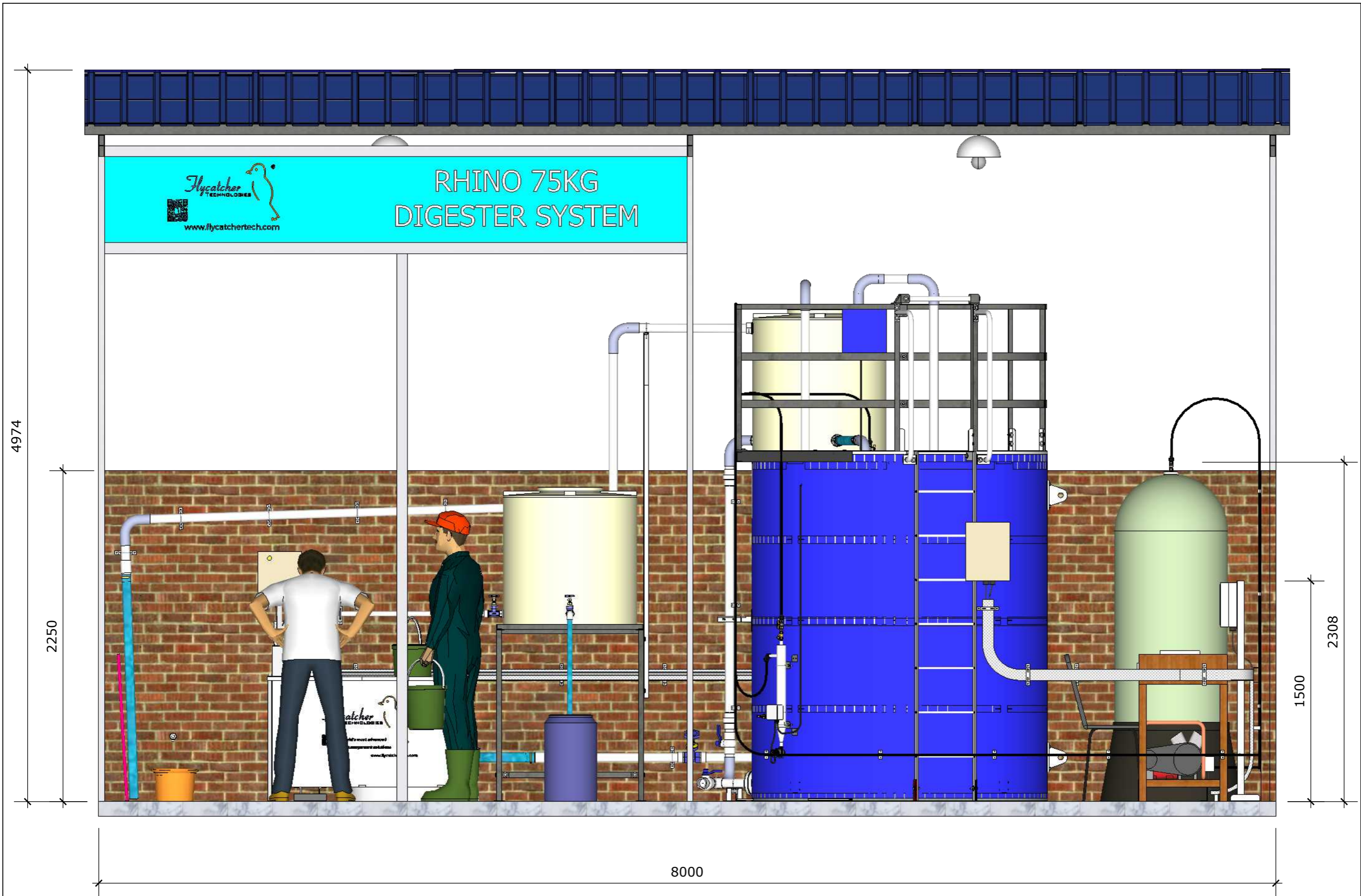
ELEVATION
